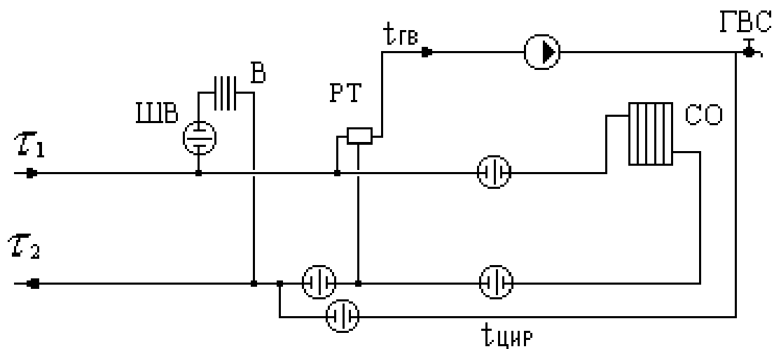
Рисунок 1 – Схема 4. Потребитель тепловой энергии с открытым водоразбором на ГВС и непосредственным присоединением СО
